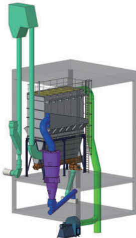
替代燃料处理系统 Alternative fuel treatment system
