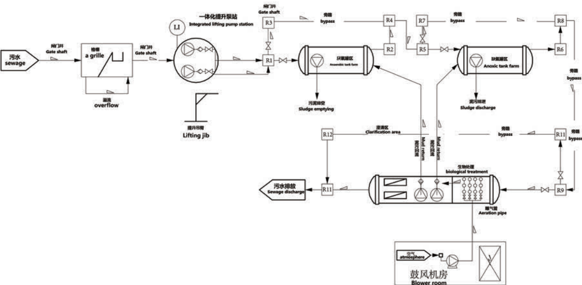
水泥厂中小型生活污水处理站工艺流程
